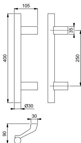
Aluminium-Stützen Edelstahl-Stange
